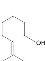
Citronelol
