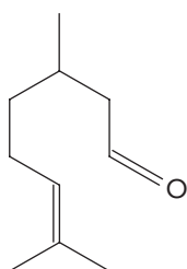
Citronelal
